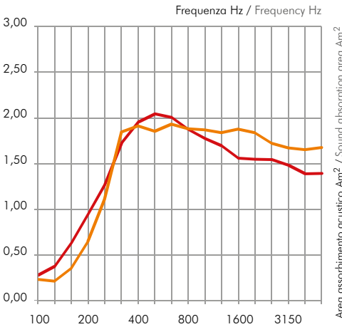
Assorbimento acustico pannello in aderenza* Adherence panel sound absorption*
